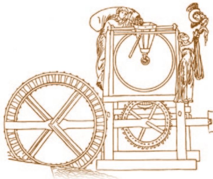
Samtidig tegning der viser pricipperne i møllen ved Gjelå
